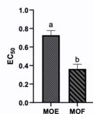
2,2-Diphenyl-1-picrylhydrazyl (DPPH)
